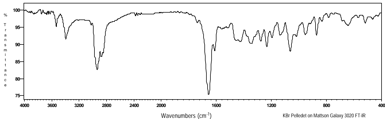
FT-IR
