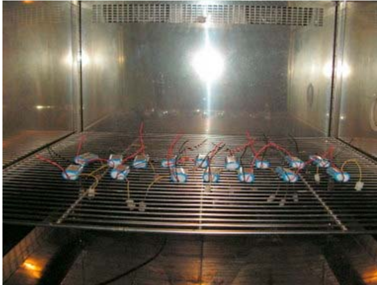
Fig.2 : Thermal test
